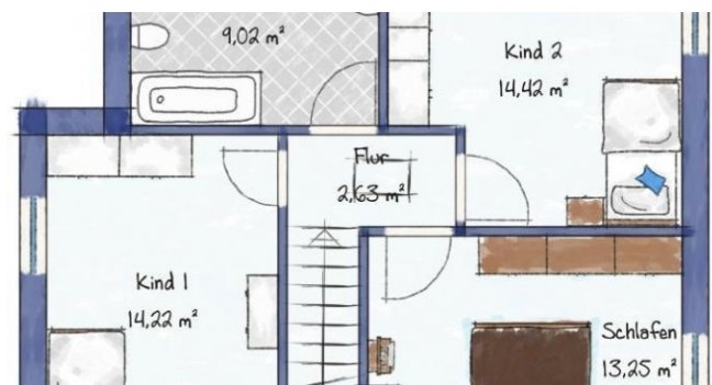
Obergeschoss
